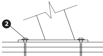
1) Tirafondo 5/16" x 2 1/2" + arandela + tarugo plástico Ø10 2) Tirafondo 5/16" x 2 1/2" + arandela
