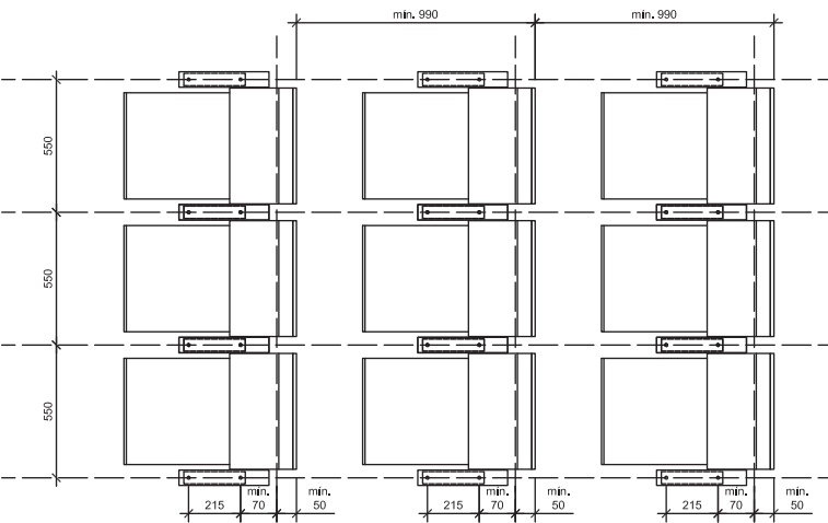
Detalle de fijación standard sobre concreto.
